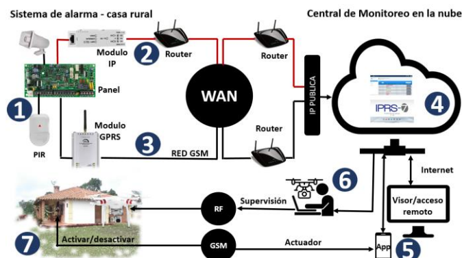
Fig. 9. Prototipo implementado para validar el modelo propuesto. Fuente: Los autores.
