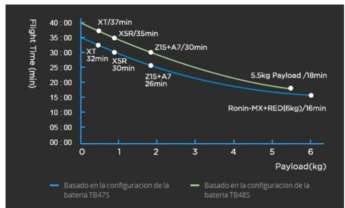
Fig. 7. Tiempo de vuelo ampliado. Fuente: [9]
